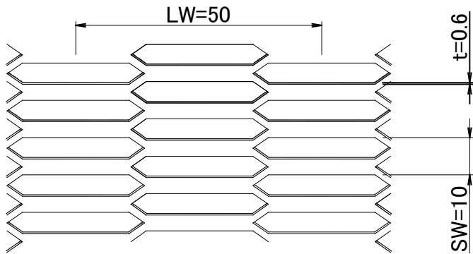
鋼製有孔型枠(ブラインド加工鋼板)詳細図
