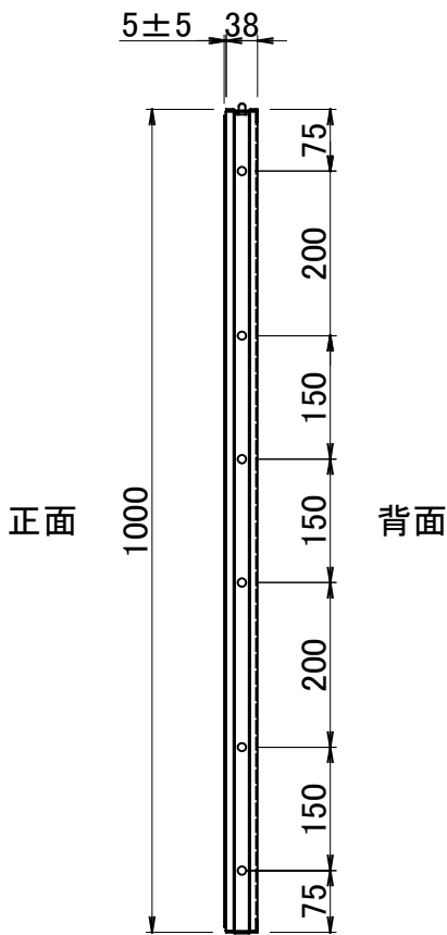
側面図
