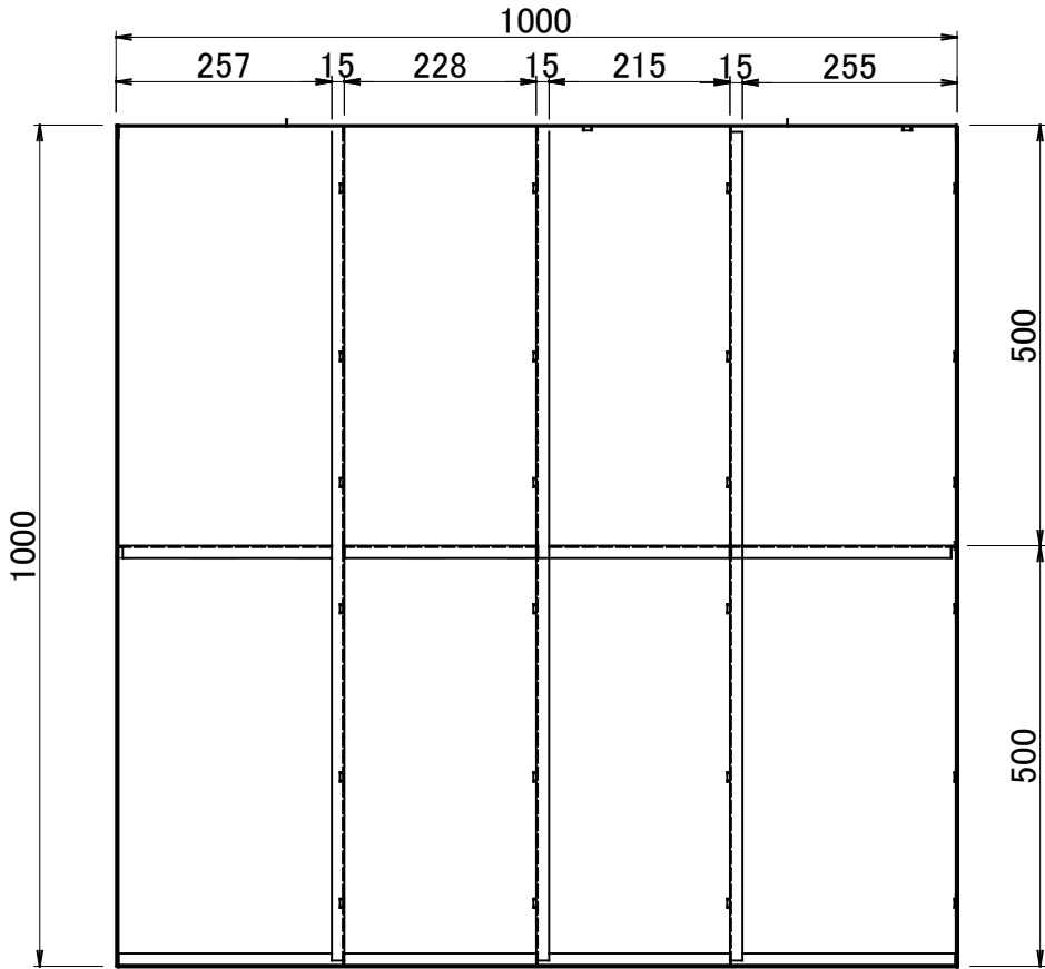
背面図
