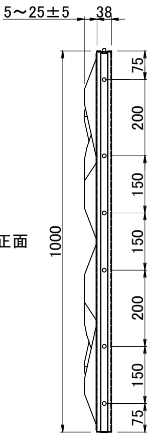
側面図
