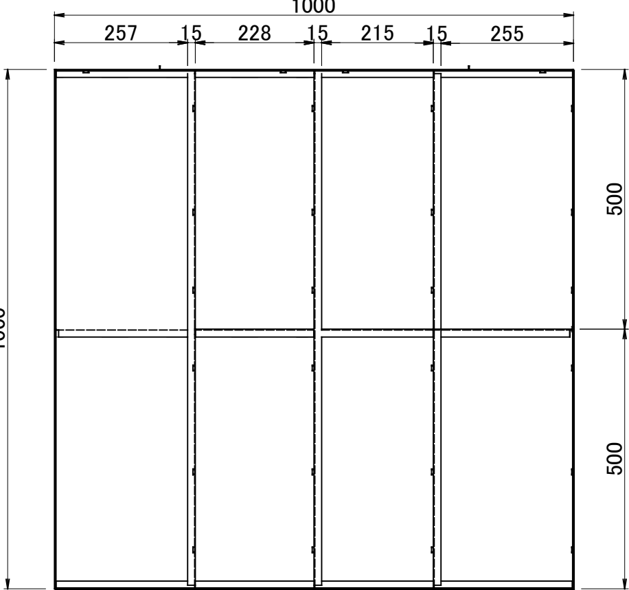
背面図
