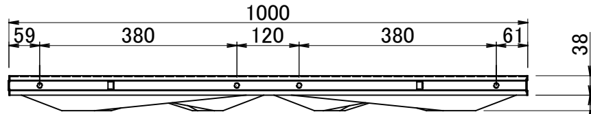
上面図
