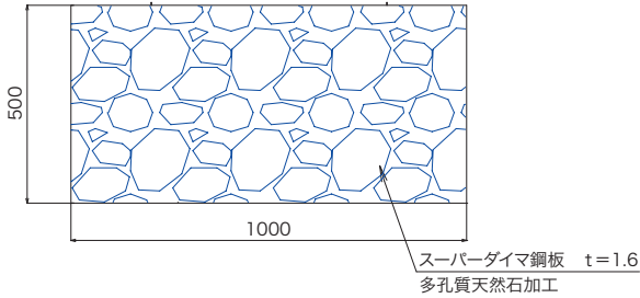
底面図
