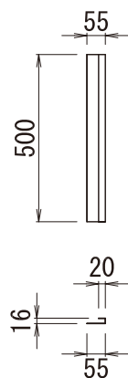
端部用カバー t = 0.6
