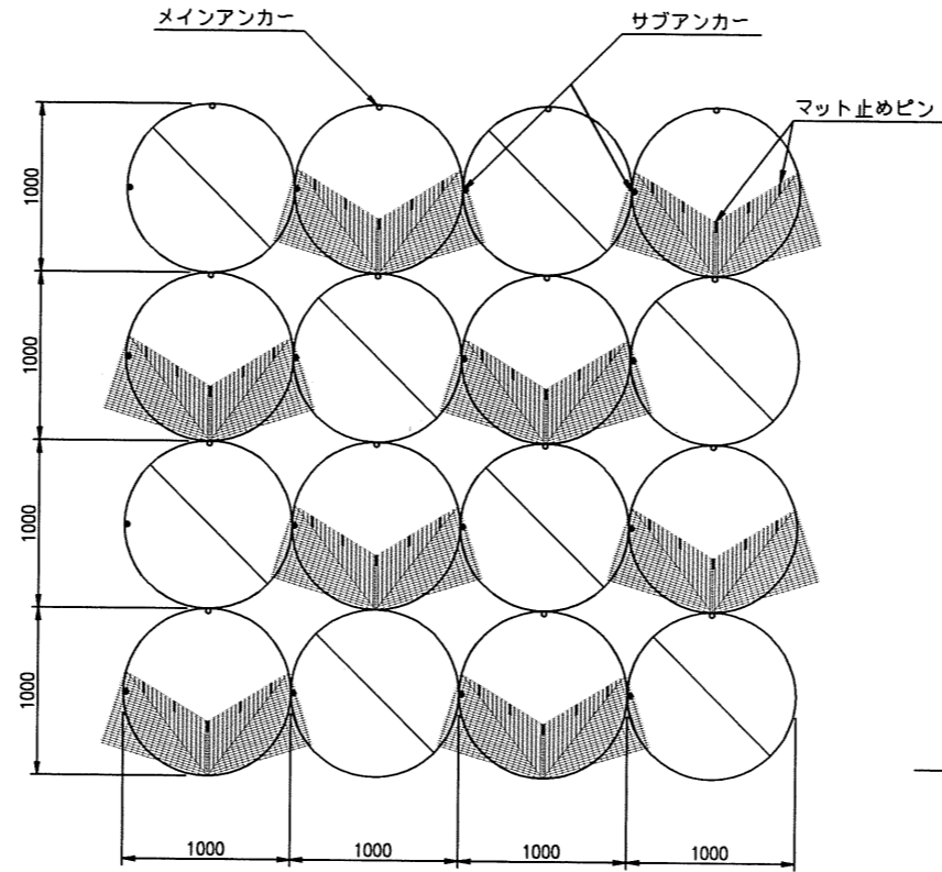
配置図 S=1/25
