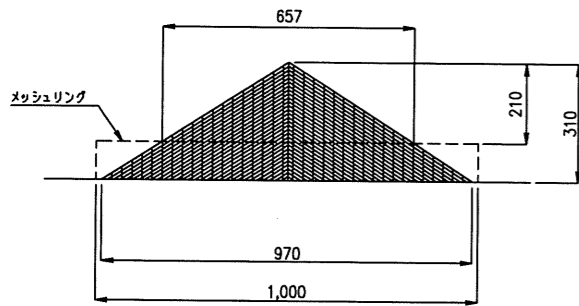
正面図 S=1/10
