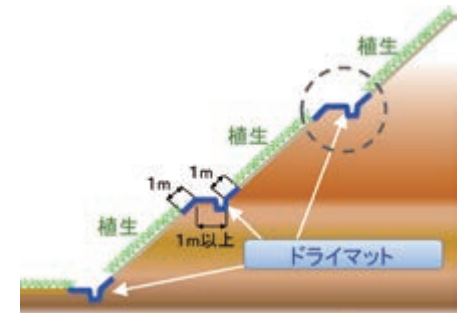
法面の施工例①
